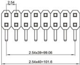
Terminal(Du Pont2.54)
