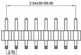
Du Pont2.54-PT
