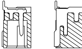
剖面 A-A
