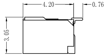
剖面 A-A
