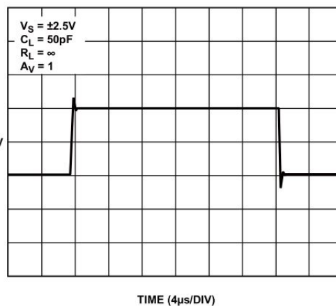
图 15. 小信号瞬态响应
