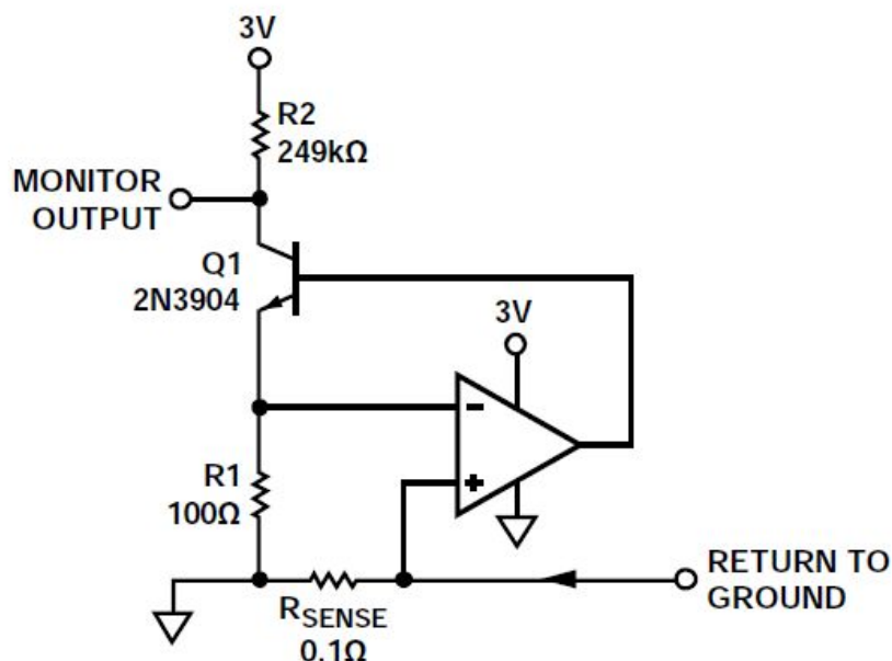
低端电流监控
