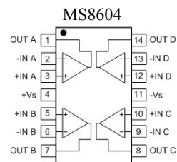
图3. 14引脚SOP14和14引脚TSSOP14
