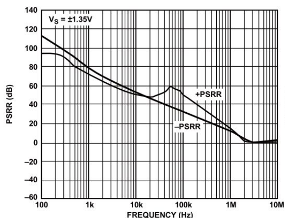
图 18. PSRR 与频率的关系
