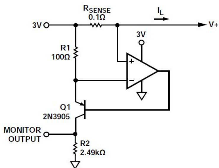
高端电流监控
