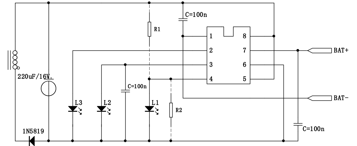
TC3582BB 典型应用方案：二灯、三灯模式，R1、R2 可选装。
