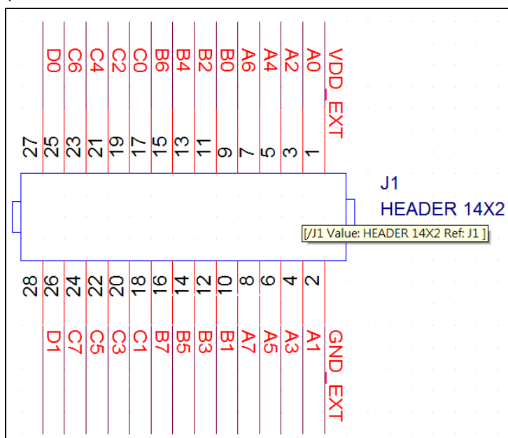
图十一、J1 接线原理图
