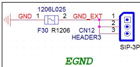
图四、CN12 接线原理图
