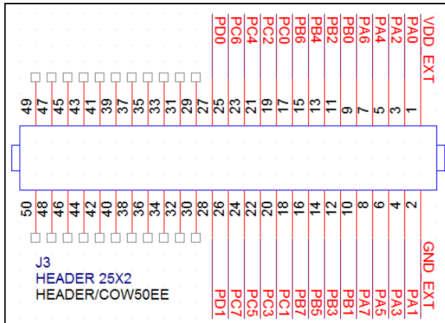
图六、J3 接线原理图
