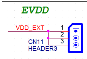
图三、CN11 接线原理图
