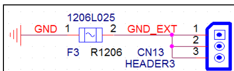
图五、CN13 接线原理图
