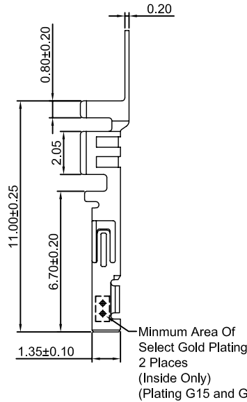
SEC:A-A
