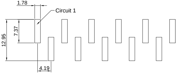
P.C.B LAYOUT
