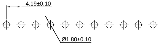
P.C.B LAYOUT
