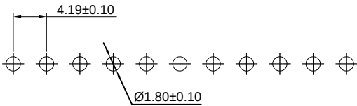
P.C.B LAYOUT
