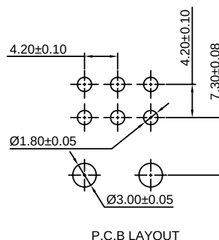
P.C.B LAYOUT
