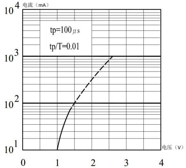
集电极电流与电压关系
