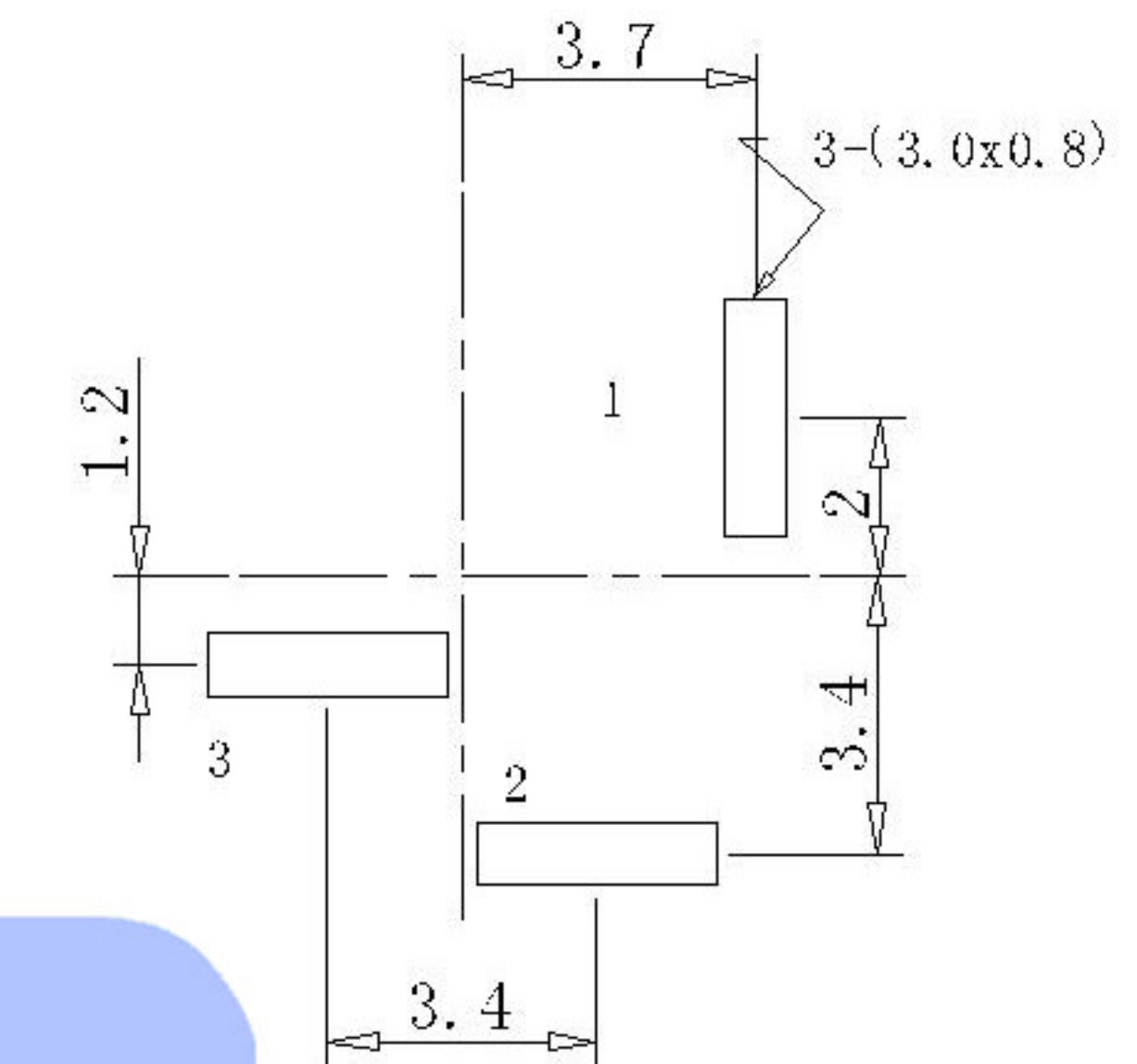
P.C.B LAYOUT
