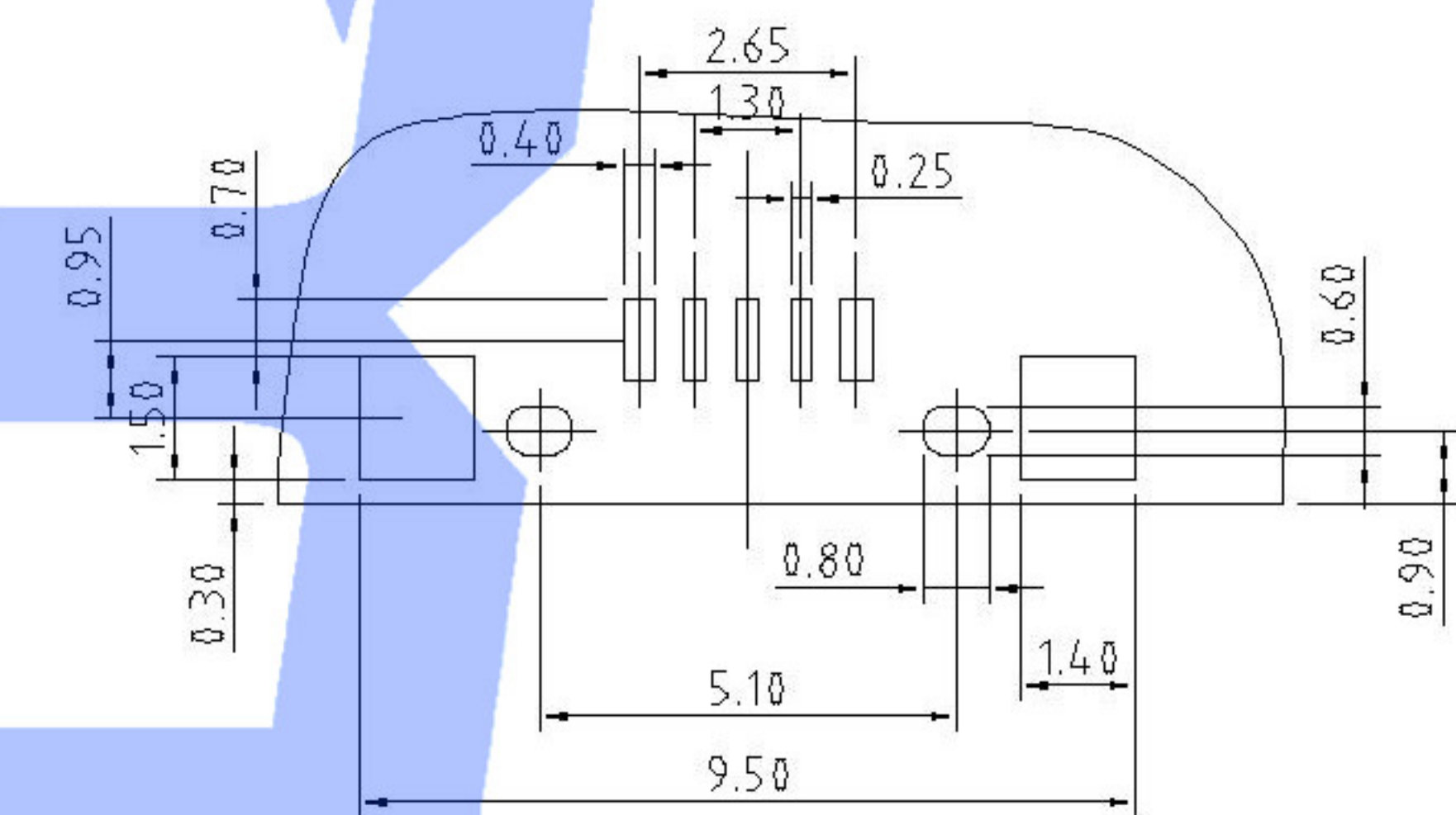
P.C.B LAYOUT
