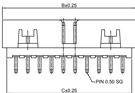
2x7P~2x25P
