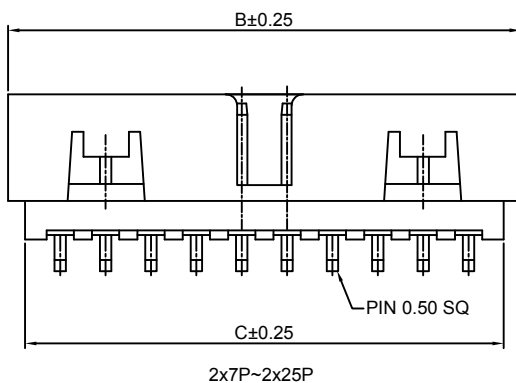
2x7P~2x25P
