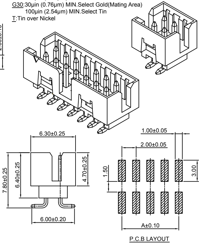
P.C.B LAYOUT
