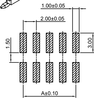
P.C.B LAYOUT
