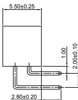
P.C.B LAYOUT
