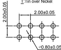
P.C.B LAYOUT
