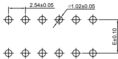
P.C.B LAYOUT
