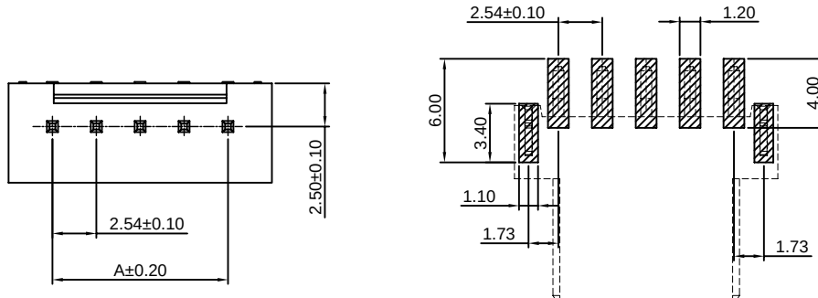
P.C.B LAYOUT
