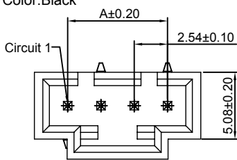
4P~25P
