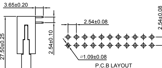
P.C.B LAYOUT
