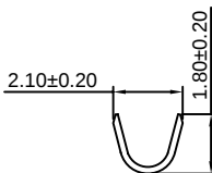
SEC:A-A
