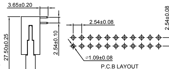
P.C.B LAYOUT
