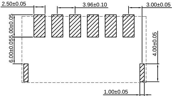
P.C.B LAYOUT
