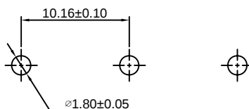
P.C.B LAYOUT
