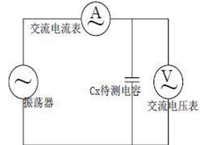
图 3. 交流阻抗测试电路图
