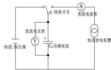
图 1. 容量测试电路
