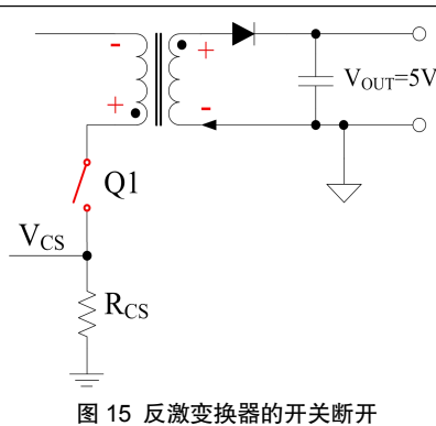
图 15 反激变换器的开关断开
