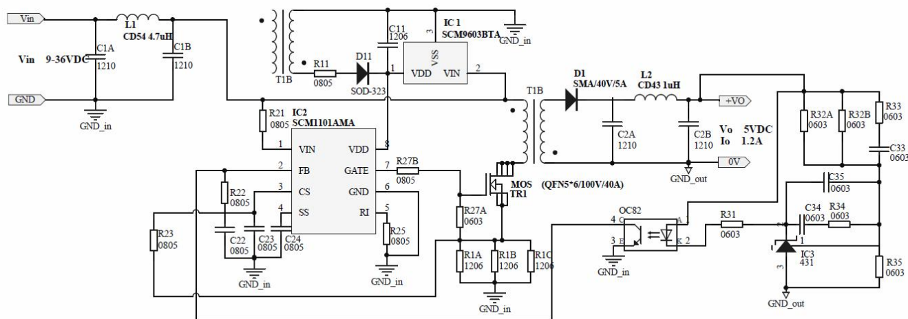
图 20 应用电路
