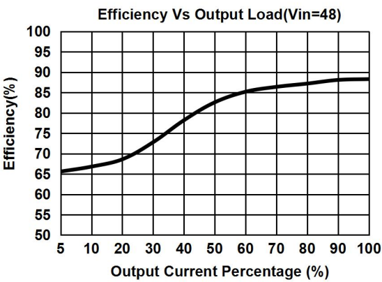
注: 该功能曲线是在 18~75V 输入、15V 双路输出的 10W 样机, 标称输入下实测得到的。
