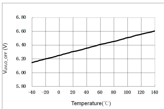
图 2 欠压锁定撤销 VS 温度
