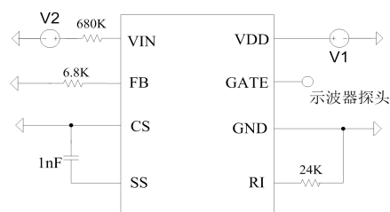
图 13 电学特性测试电路原理图
