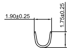
SEC:B-B
