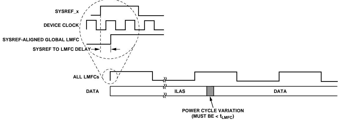
Figure 122. SYSREF_x and LMFC
