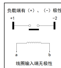
端子配置/内部连接图
