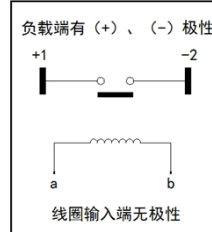
端子配置/内部连接图
