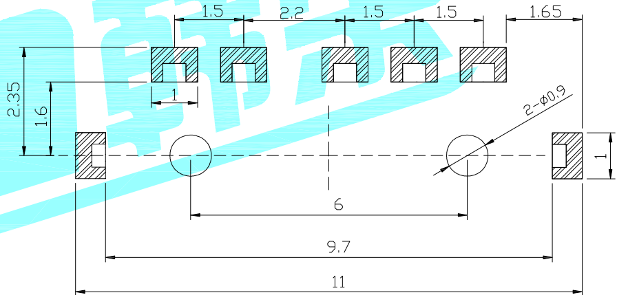
P.C.B layout
