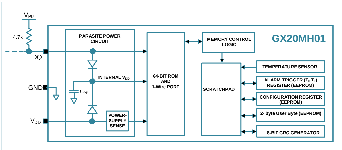
图 1. GX20MH01 的结构框图
