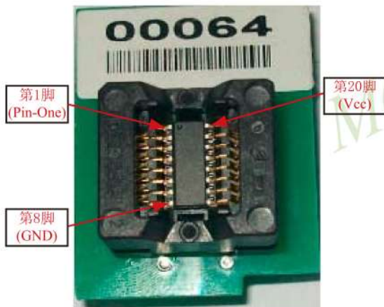
SOP-16封装的单片机安装图
