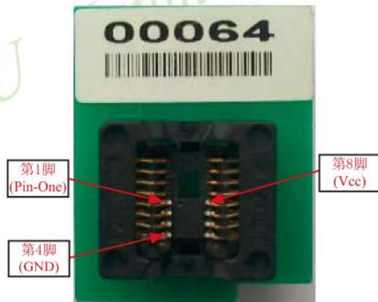
SOP-8封装的单片机安装图
