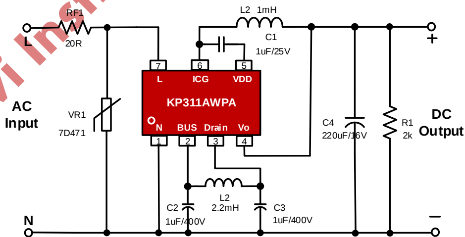
图 1 典型应用电路图
