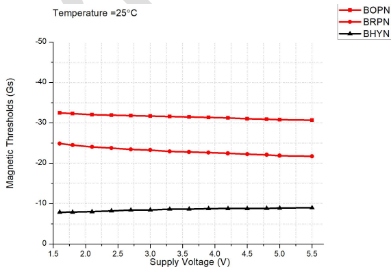
磁场阈值 vs. 供电电压 @ T_A=25^\circ\text{C}
