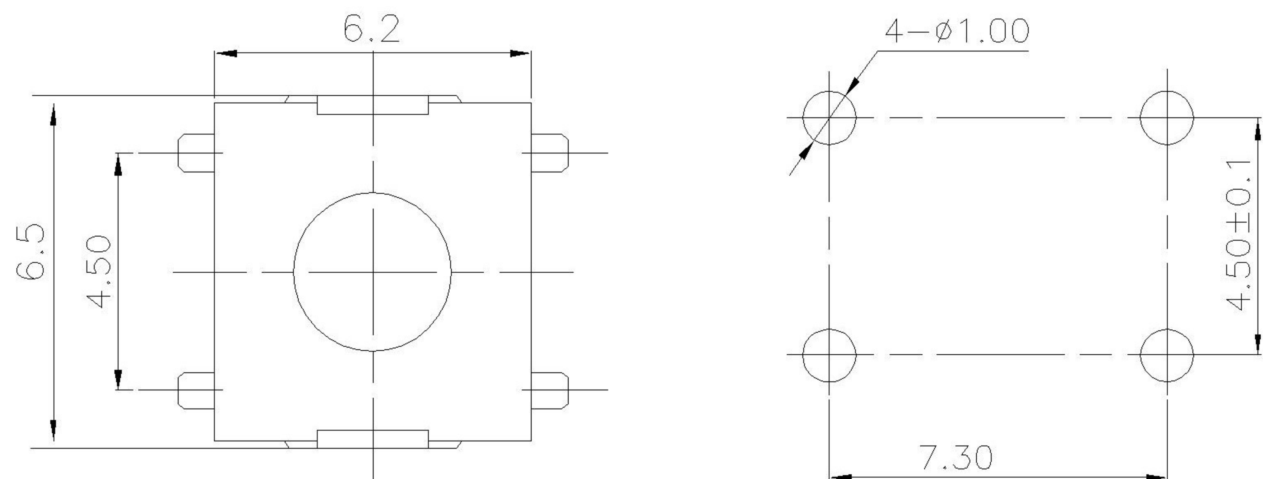
PCB Layout(Pattern side)
