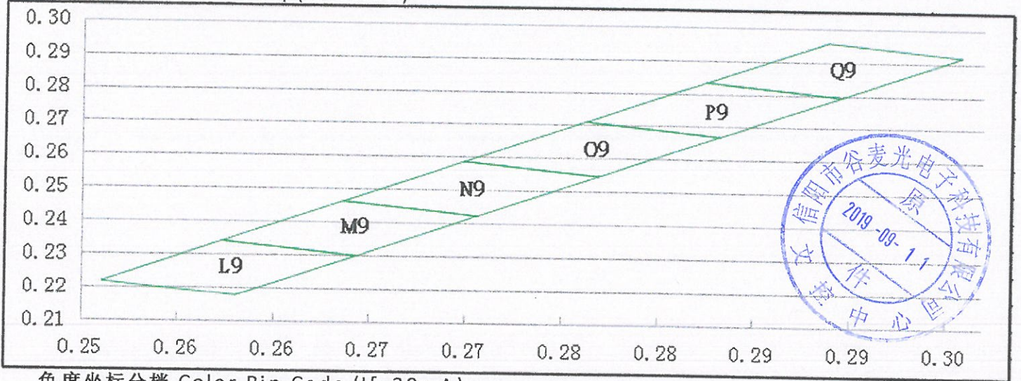
色度坐标分档 Color Bin Code (I f =20mA)
