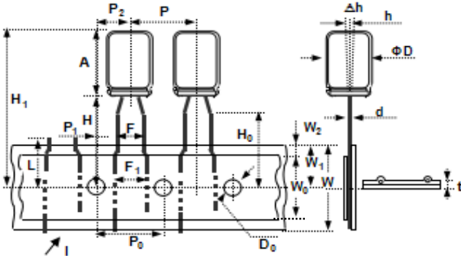
[ Fig. 4 (Diameter for Φ10、Φ13、Φ16]
