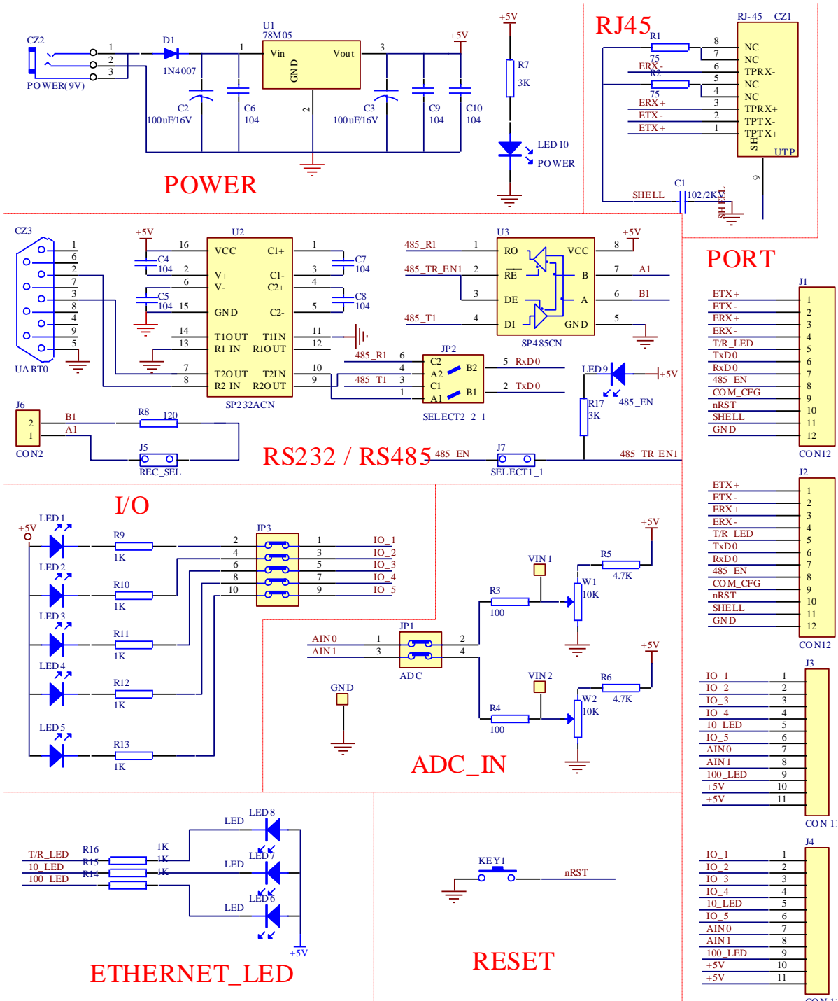
图 2.10 ZNE 评估板原理图
