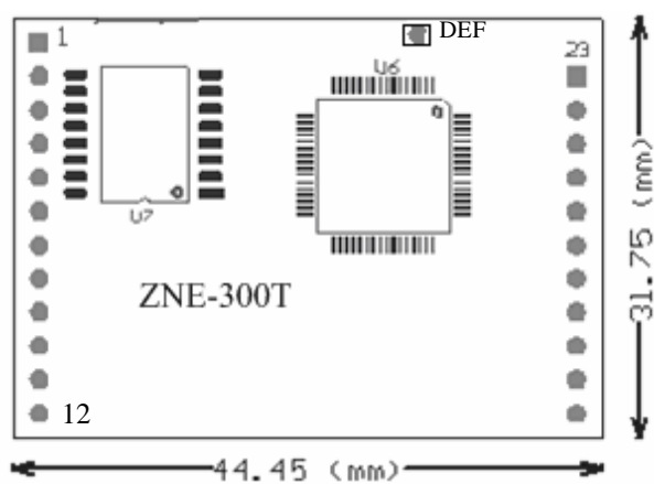
图 5.14 恢复出厂设置的跳线位置
