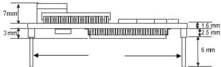
图 1.2 ZNE-300T/TI 模块侧视图及机械尺寸
