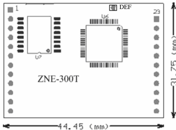
图 2.2 ZNE-300 模块俯视图及机械尺寸
