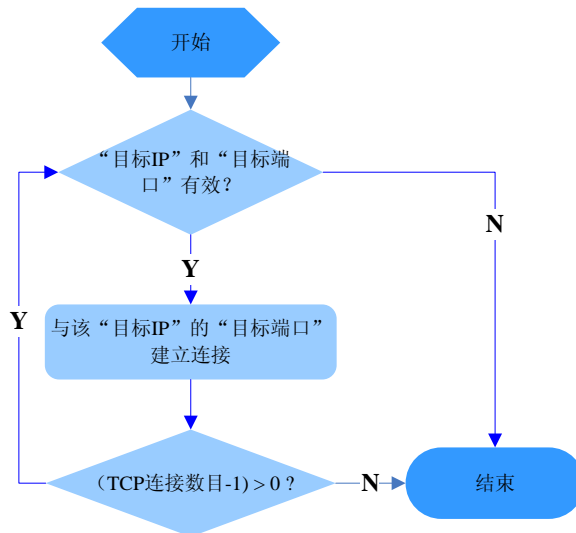
图 6.14 ZNE-300T 模块在 TCP Client 模式下建立连接流程
