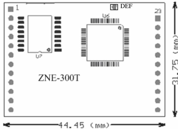
图 1.1 ZNE-300T/TI 模块俯视图及机械尺寸
