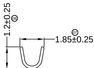
SECTION: B-B SCALE: 1:1
