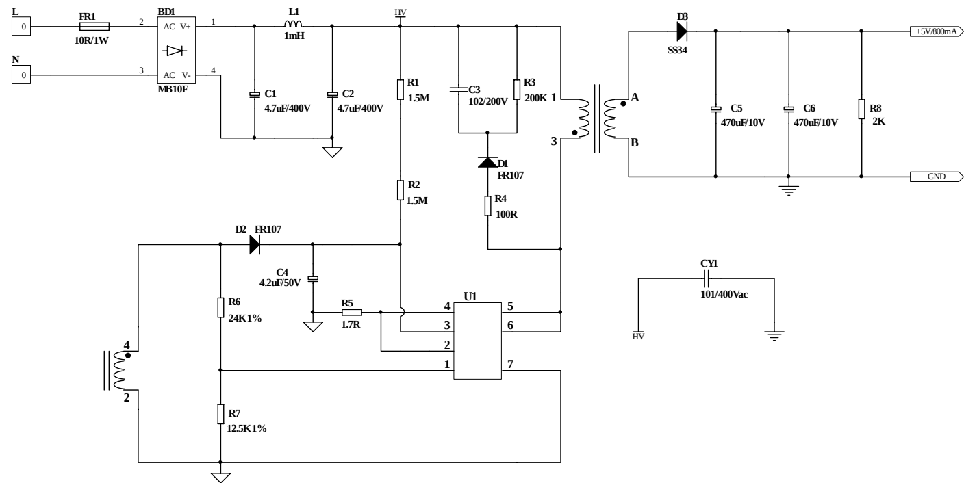
典型应用电路图
