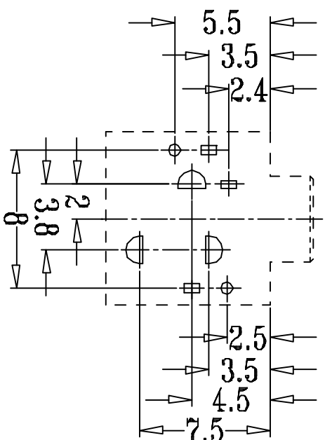
P.C.B LAYOUT
