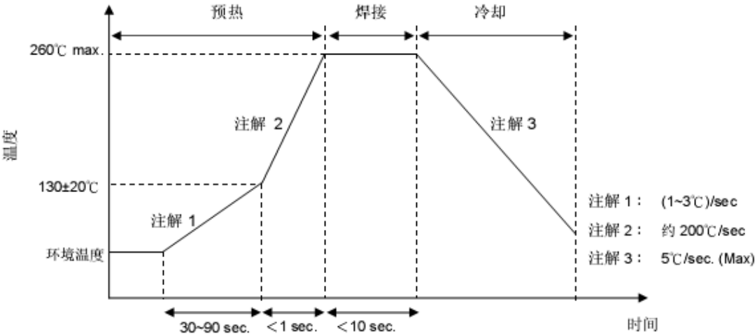
波峰焊曲线
