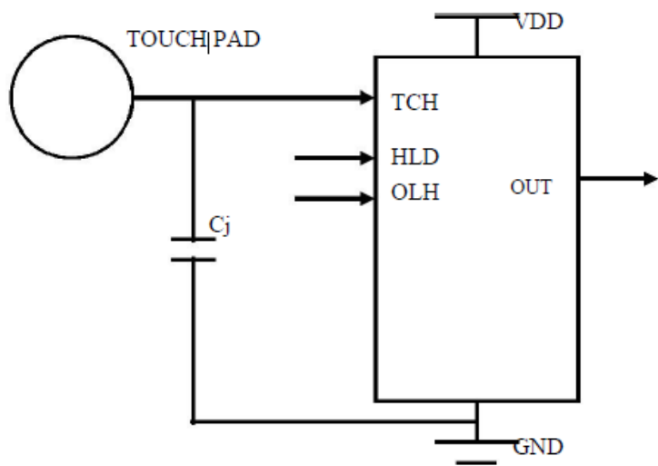
图 5 应用电路示意图
